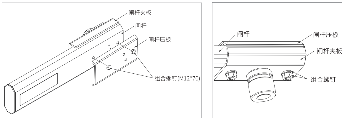
图2-2 直杆安装
