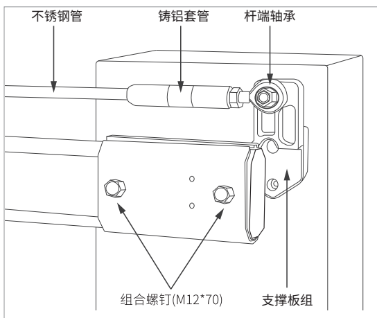
图2-3 曲臂杆安装
