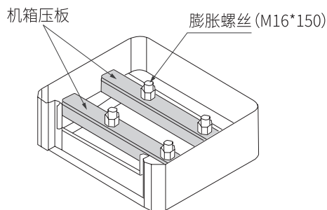
图2-1 机箱固定
